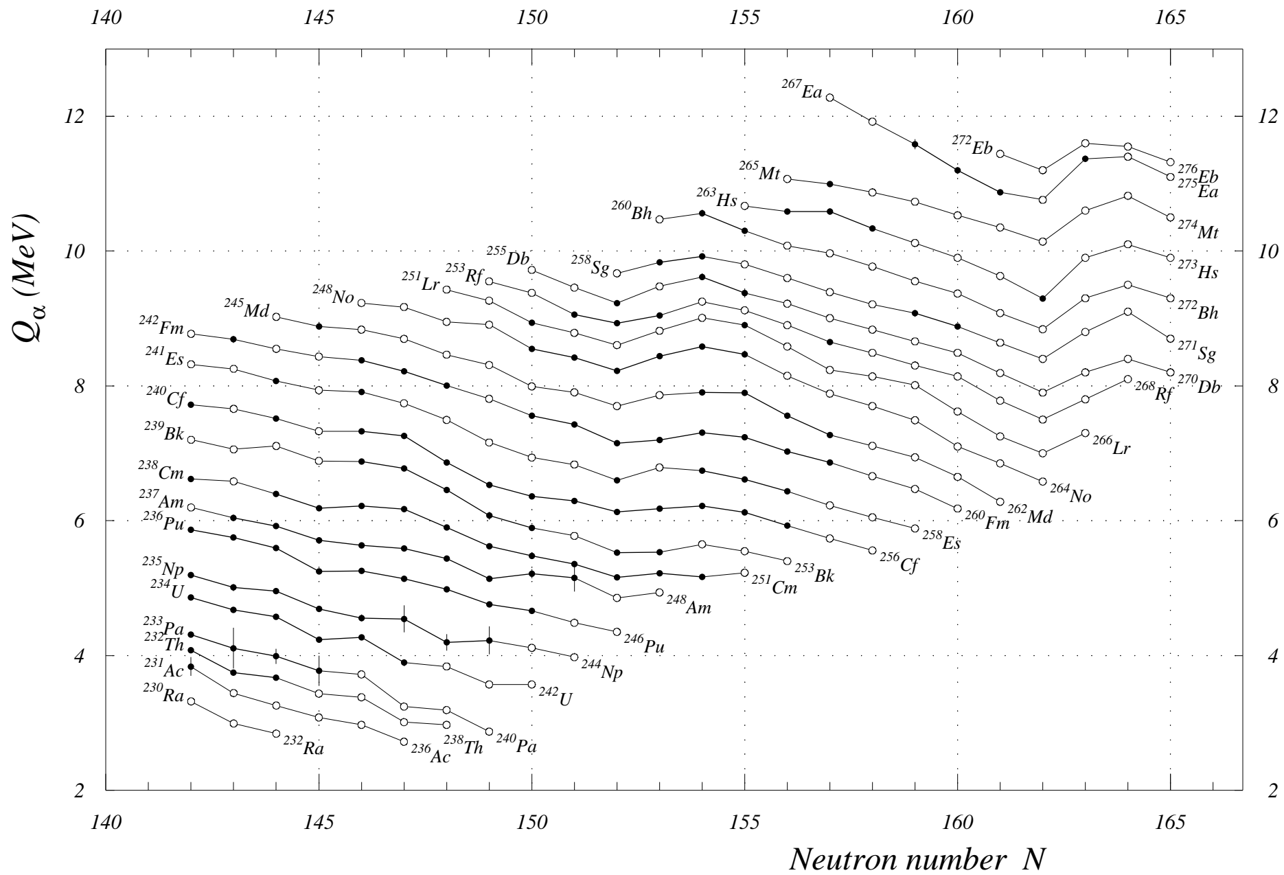
Fig. 25. \alpha -decay energies
